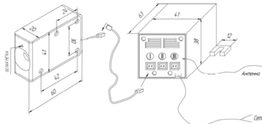
Рис. 1 Присоединительная схема замка
